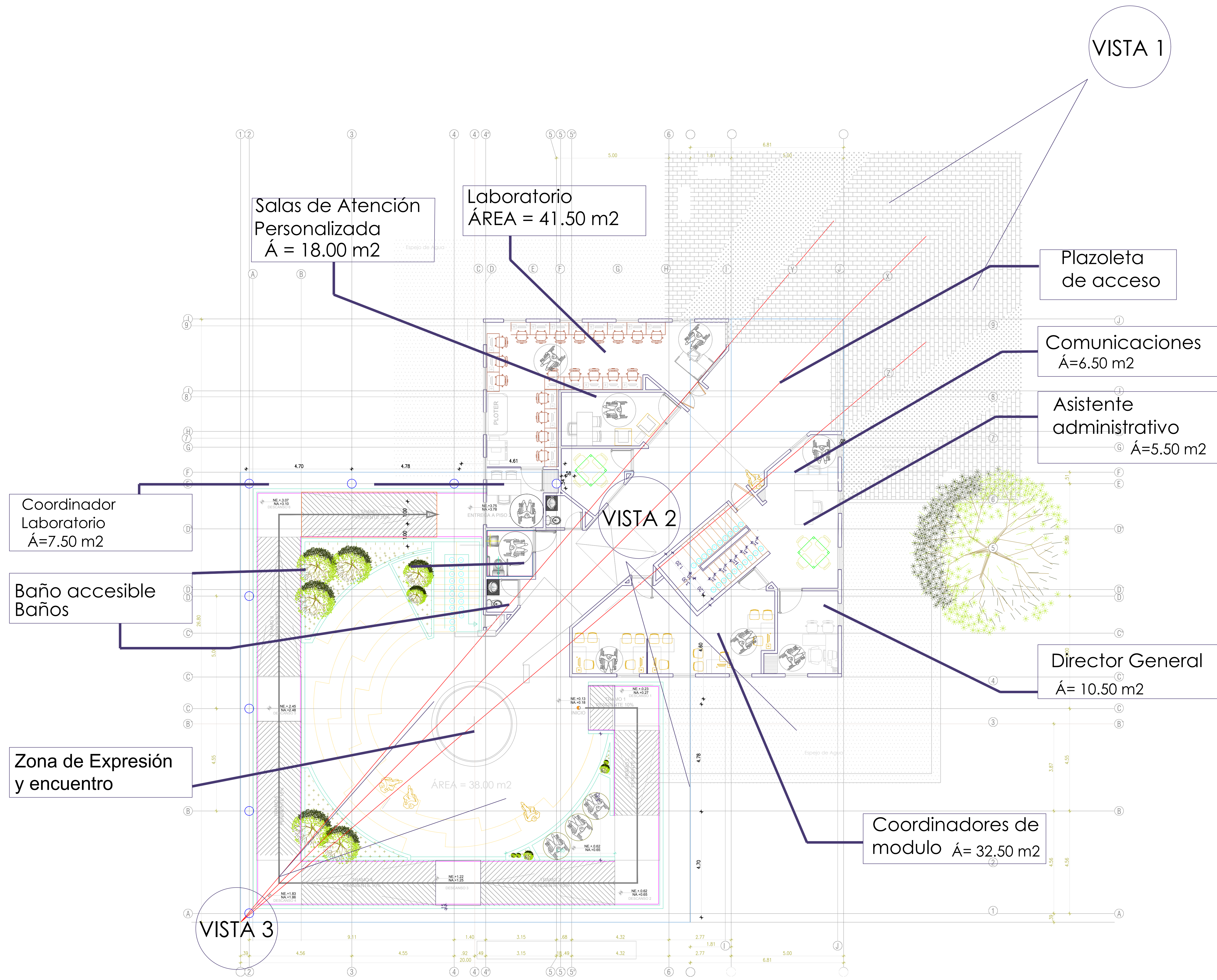
PLANTA PRIMER PISO Esc. 1:75
